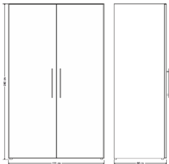
Skizze: SKM - Maße
