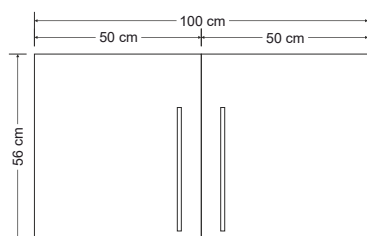
HS 100 - Skizze
