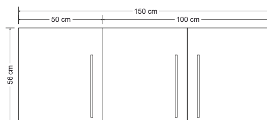
HS 150 - Skizze
